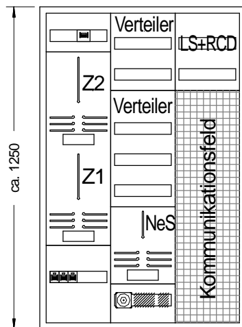
Einkundenanlage mit PV-Anlage und Kommunikationsfeld
